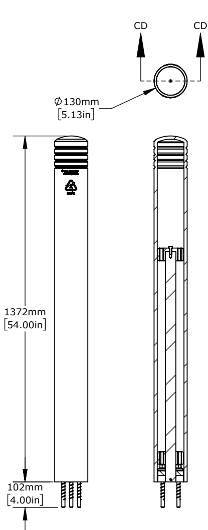
SECTION CD-CD
